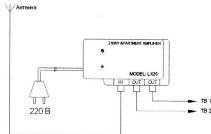
Схема подключения усилителя LX-20
